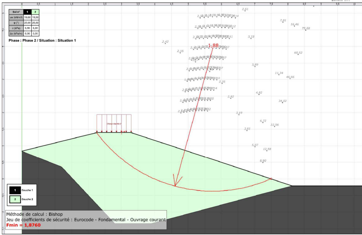
Résultat de calcul de stabilité en phase provisoire avec le logiciel TALREN
