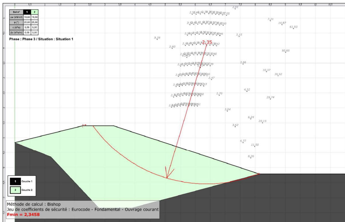
Résultat de calcul de stabilité en phase définitive avec le logiciel TALREN
